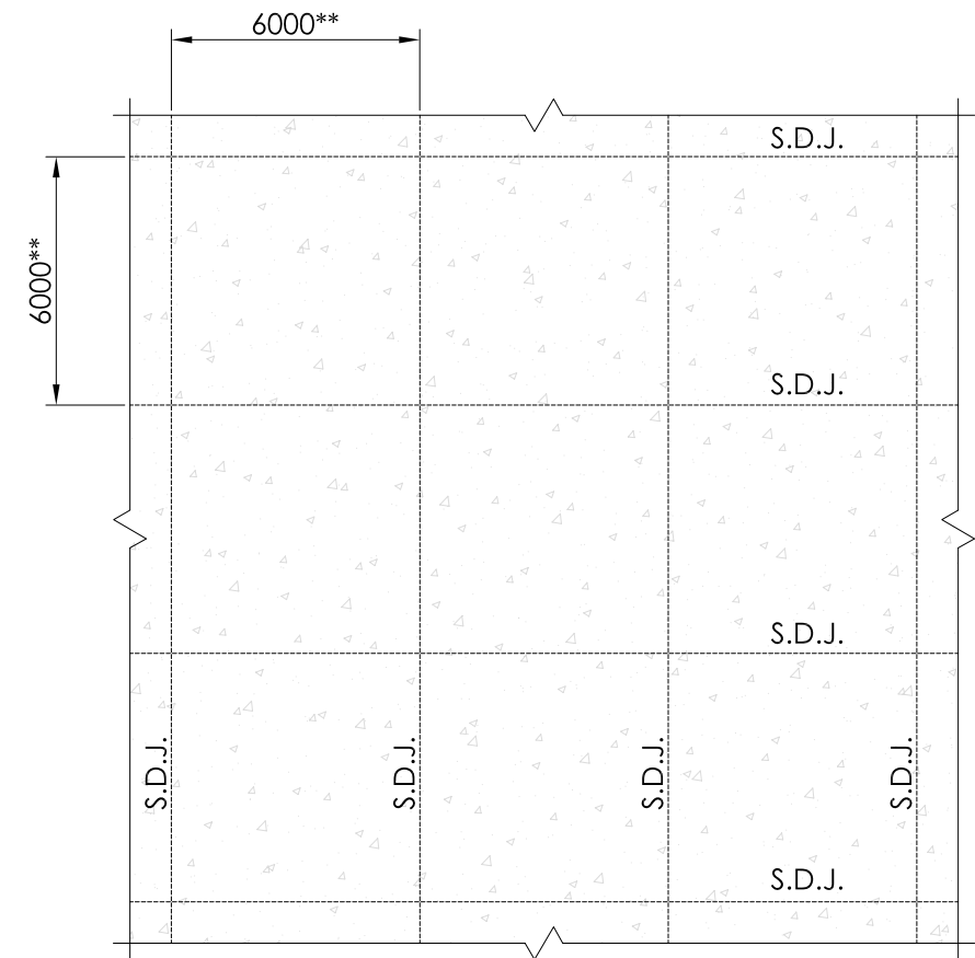
MESH REINFORCED SLAB SCALE: 1:200
