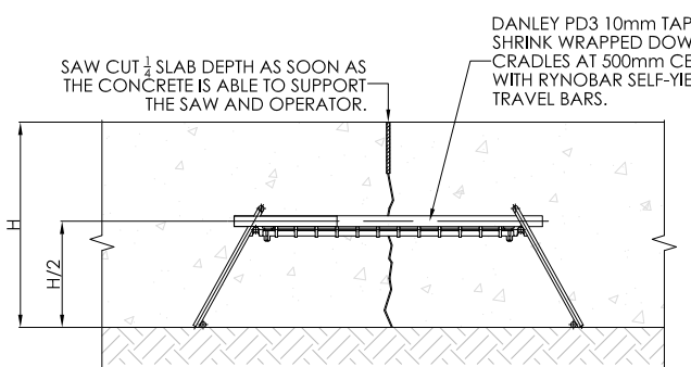
SAWN DOWEL JOINT (S.D.J.) SCALE: 1:8
