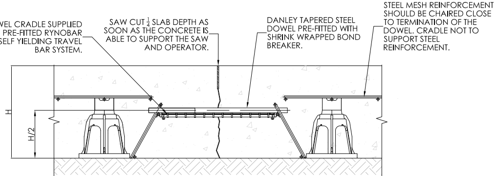
SAWN DOWEL JOINT (S.D.J.) SCALE: 1:8
